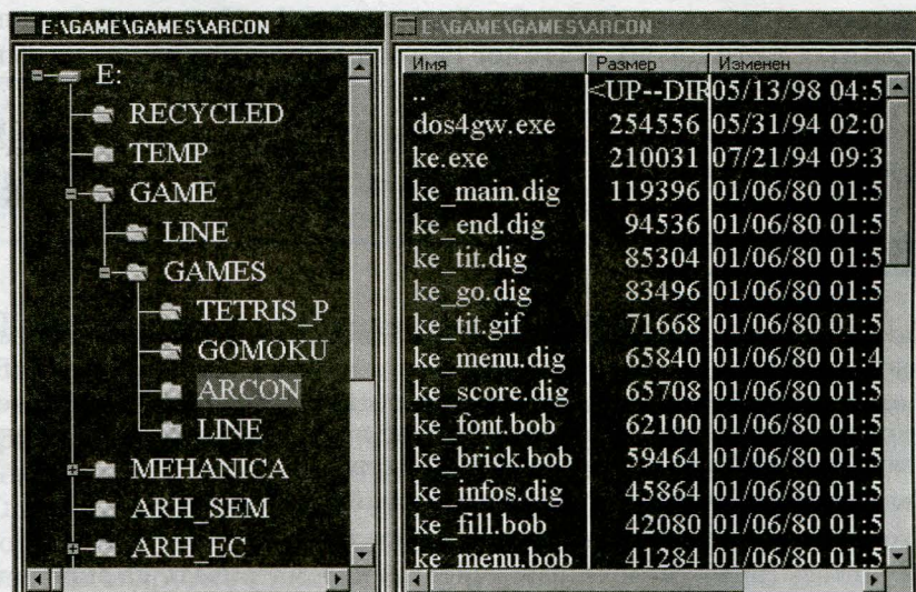
Рис. 2.11. Дерево каталогов
