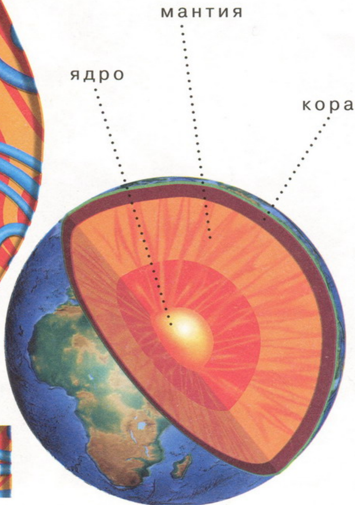
строение Земли
